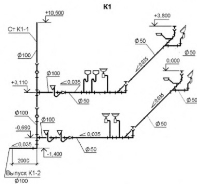
Рисунок Б.2 — Пример выполнения схем систем канализации
