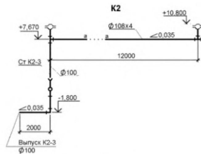
Рисунок Б.2 — Пример выполнения схем систем канализации
