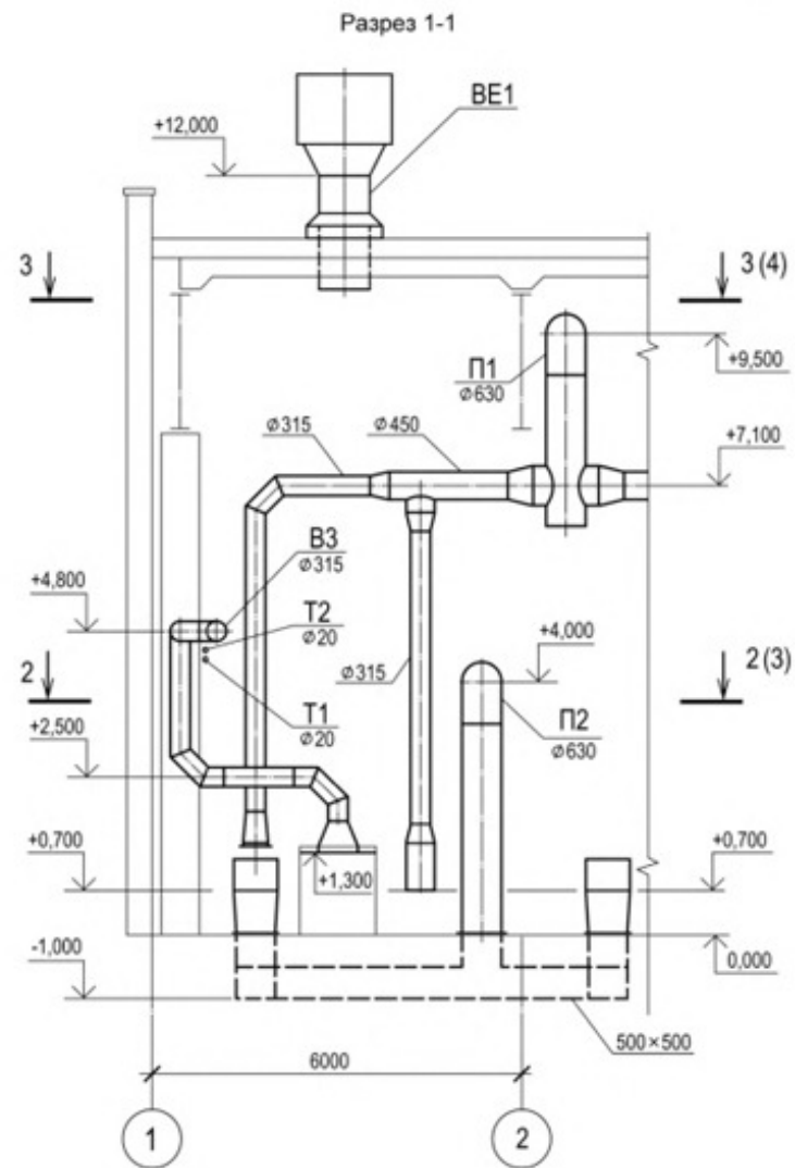
Рисунок Б.3 — Пример выполнения разреза систем
