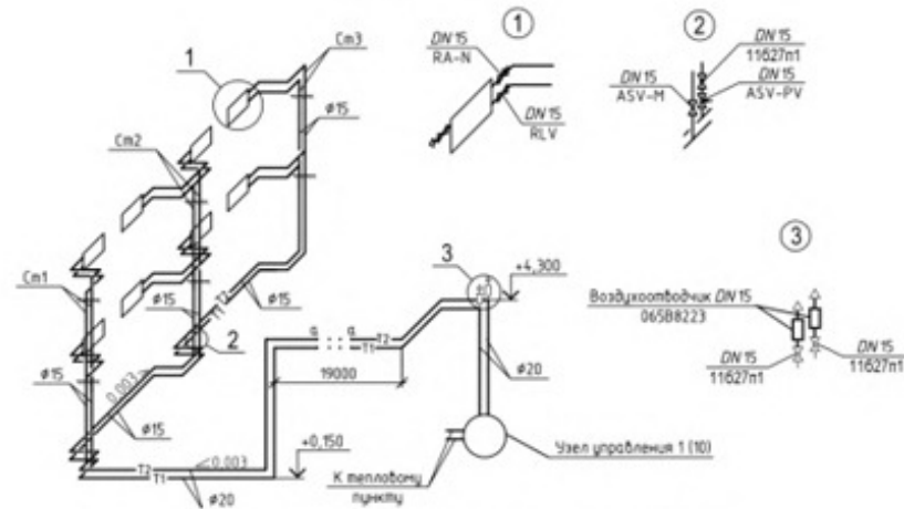
Рисунок В.1 — Пример выполнения схемы системы отопления
